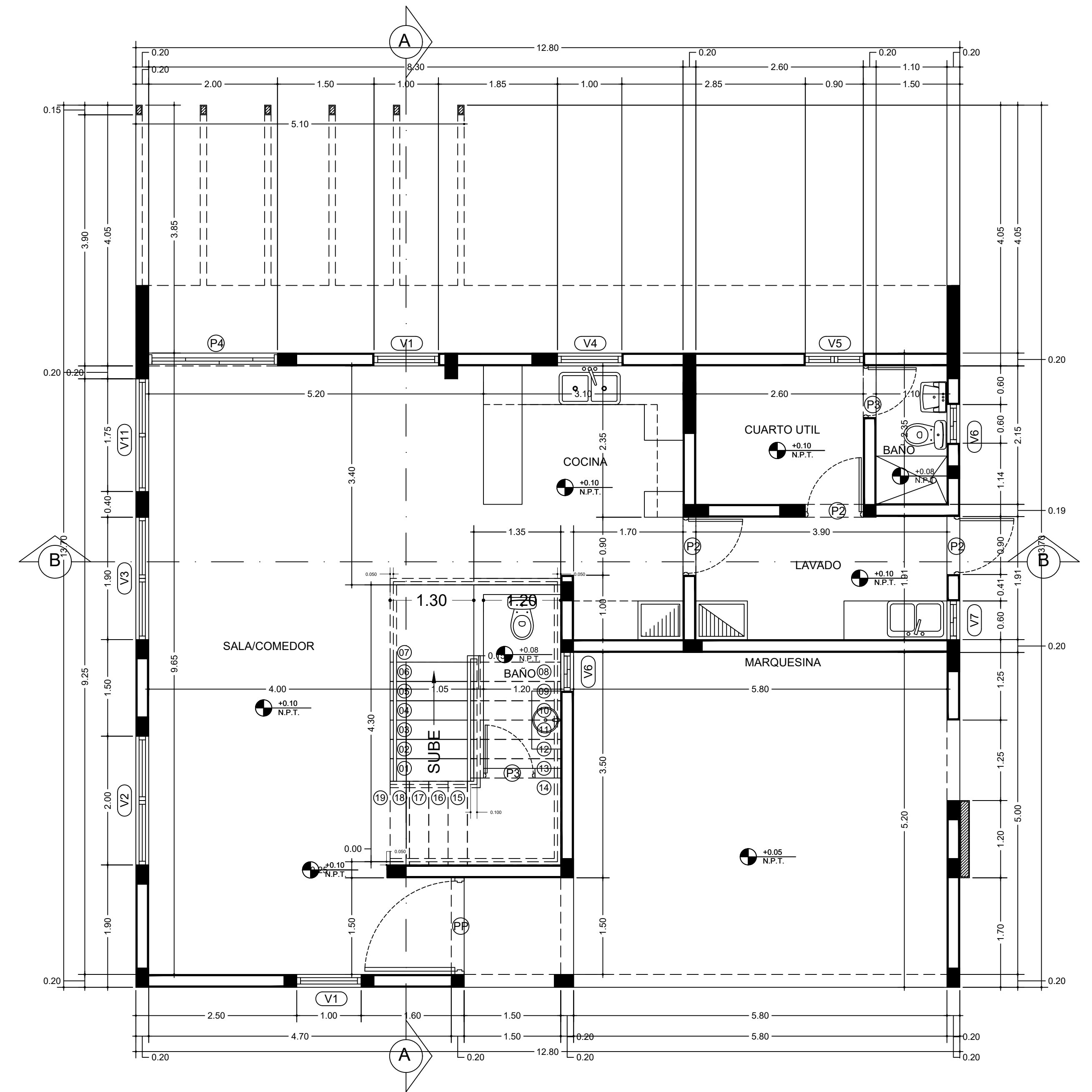
PLANTA ARQUITECTONICA DIMENSIONADA 1ER NIVEL - Esc. 1:50
