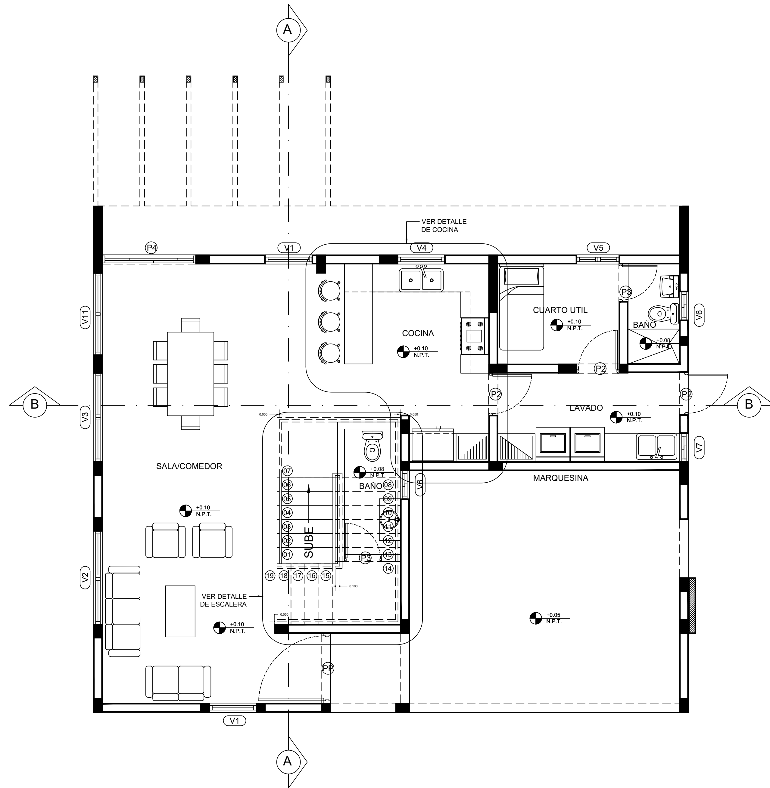
PLANTA ARQUITECTONICA AMUEBLADA 1ER NIVEL - Esc. 1:50
